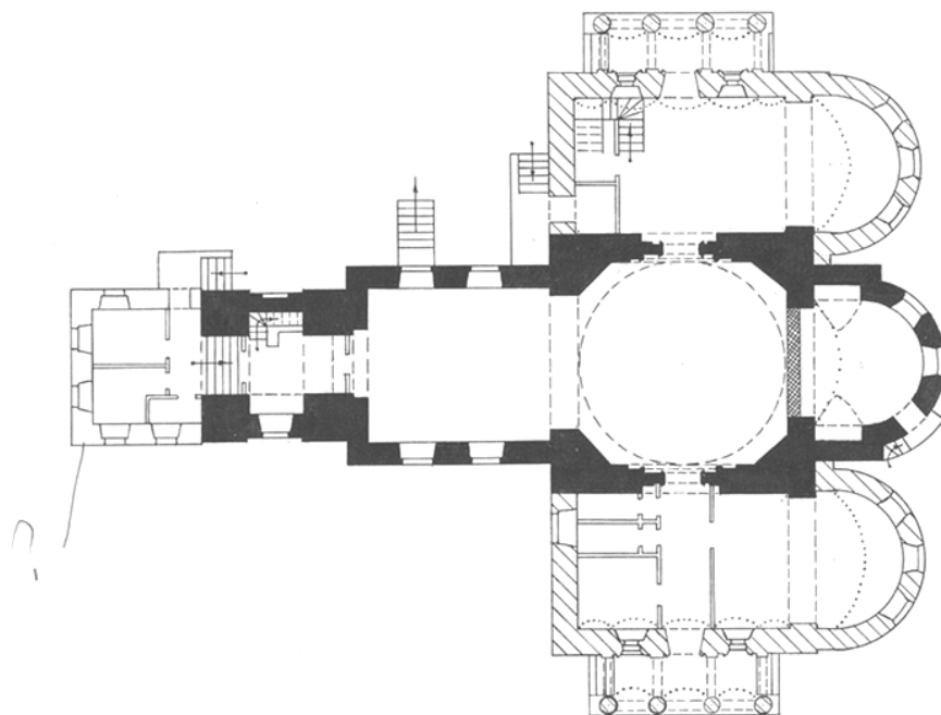
Церковь Владимирской иконы Божией Матери, 1831-1833 гг., 1894-1895 гг., план
