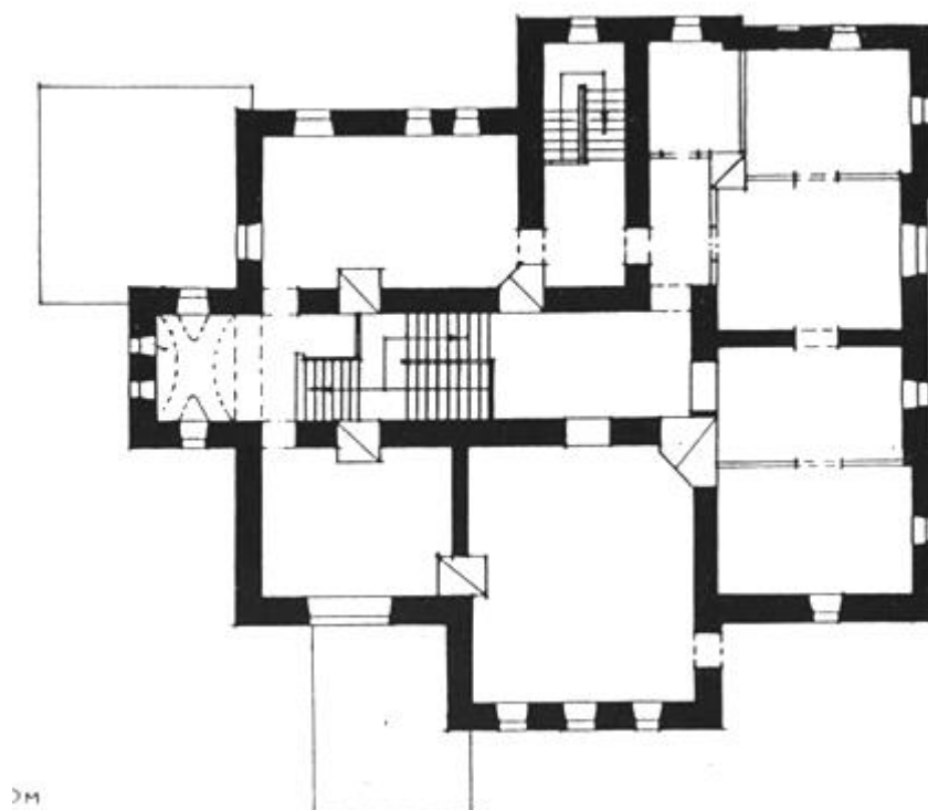
Дача писателя Телешова Николая Дмитриевича, план 2-го этажа
