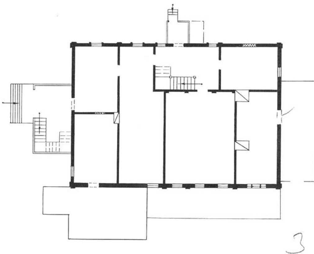
Усадьба "Коренево": главный дом, план 1-го этажа
